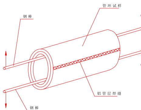
图 1 管环径向拉力试验
